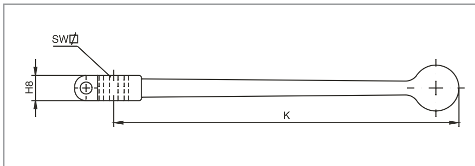
Griff gerade, Aluminium rot eloxiert
