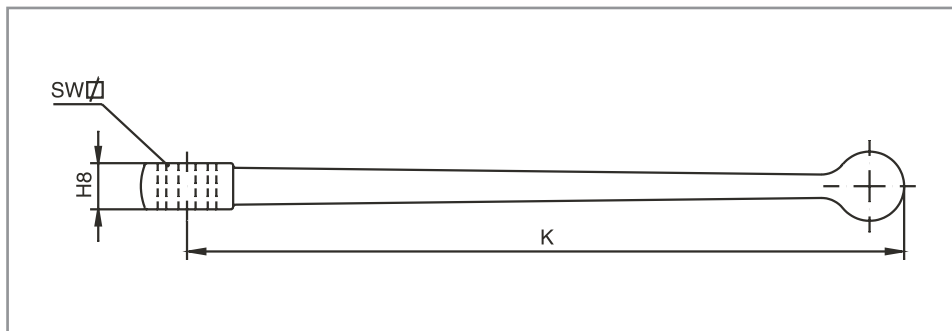
Griff gerade, Zinkdruckguss
