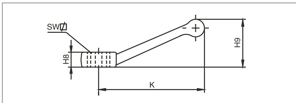
Griff gekröpft, Zinkdruckguss
