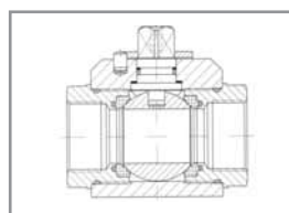
Kugelhahn mit Metalldichtungen
