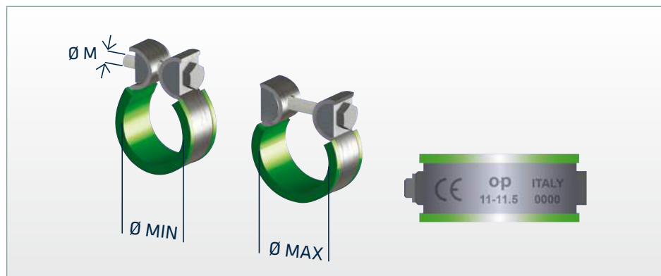
FASCETTE STOPFLEX PER TUBO FLESSIBILE
