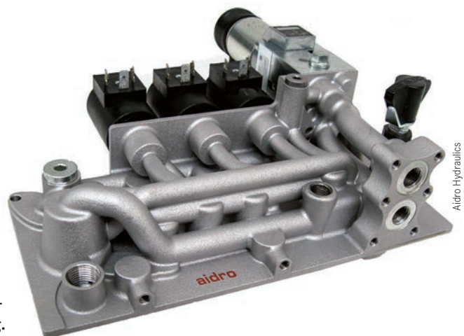
Neben strömungstechnischen Verbesserungen ermöglicht die additive Fertigung eine deutliche Gewichtsreduzierung. Die konventionell gefertigte Hydraulikkomponente (links) wiegt 5 kg, das Bauteil mit gleicher Funktion aus dem 3D-Drucker nur 1,3 kg.
