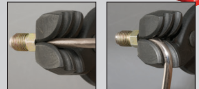
Bremsrohrzange
